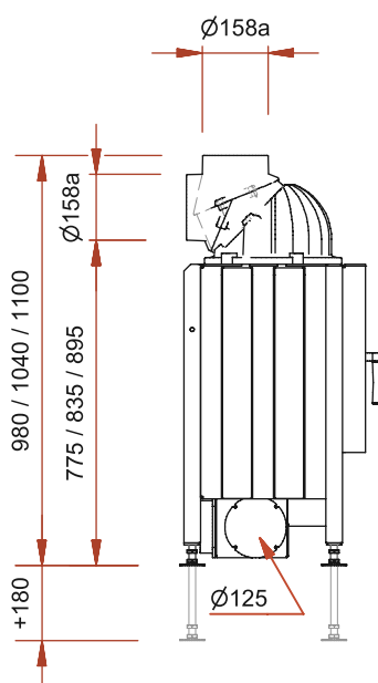
Seitenansicht M 1:20
