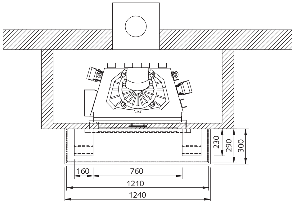
Draufsicht
