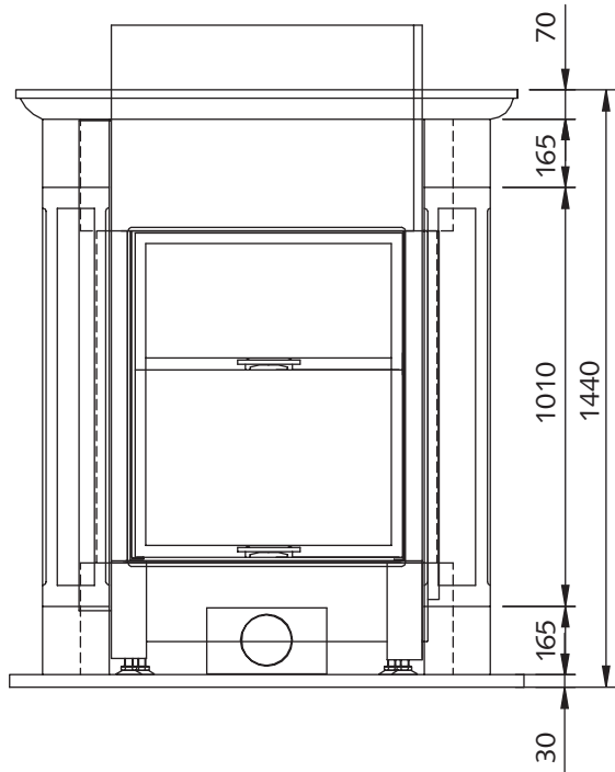
Ansicht
