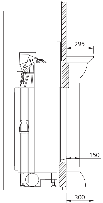
Seitenansicht
